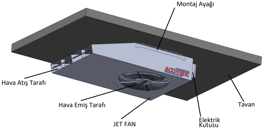
Radyal Jet Fan Tavan Montaj Detayı
