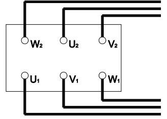
Y/Δ Bağlantı
