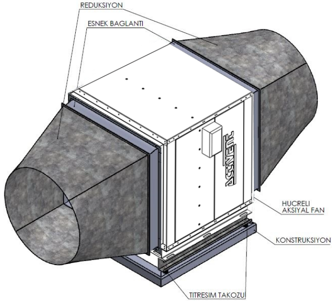
Aksiyal Hücreli Taze Hava Fanı Bağlantı Şekli
